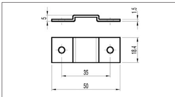
04 1218 001 000 Rúdvezető lemez központi fiókszárhoz
