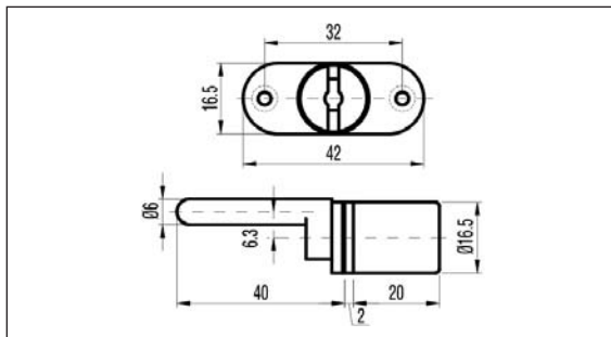
03 0922 006 004 Központi fiókszár, előről záródó
