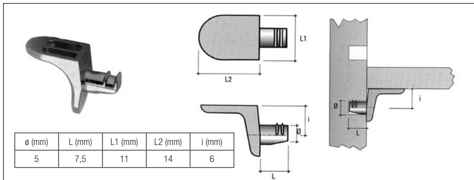
ME05 Körmos polctartó
