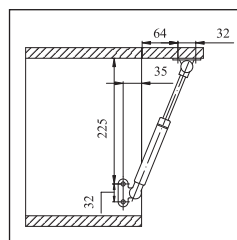
Gázteleszkópos felnyíló olló
