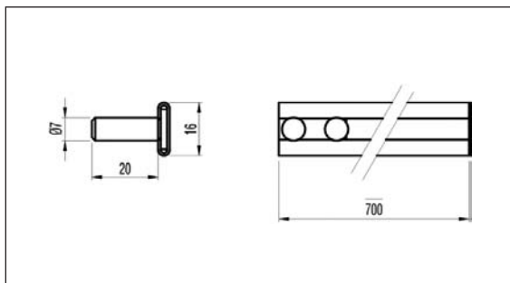
03 0922 650 C-profilú zárrúd központi fiókszárhoz
