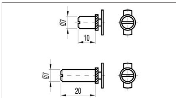
03 0912 003 Fiókrögzítő csap központi fiókszárhoz
