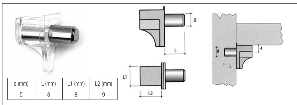
ME13 Csapos polctartó
