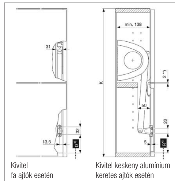
HUWILIFT Senso raktárkészlet
