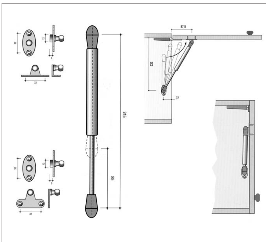
Gázteleszkópos felnyíló olló
