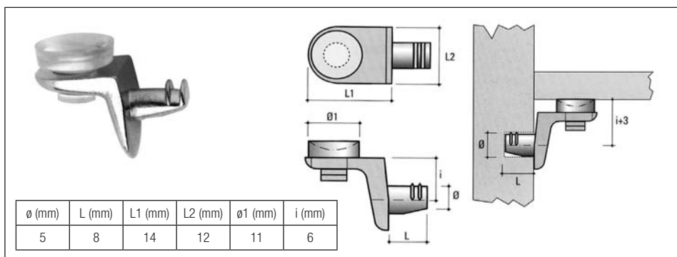
MV03 Körmos üvegpolc tartó
