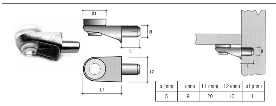
MV01 Csapos üvegpolc tartó
